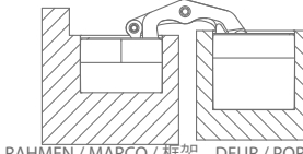
KADER / CADRE / FRAMEFrame
