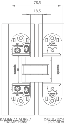
KADER / CADRE / FRAMEFrame
