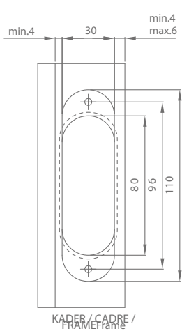
KADER / CADRE / FRAMEFrame
