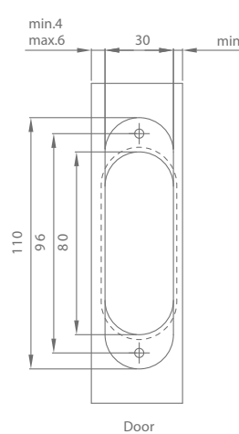
DEUR / PORTE / DOORDoor
